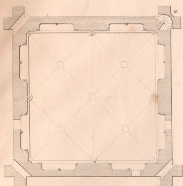
IIIter Grundriß.
